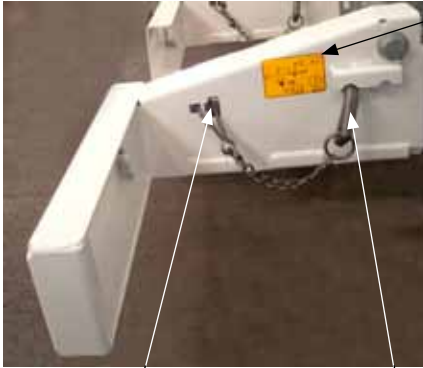
Kippstecker
